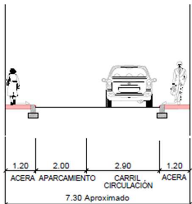
SECCIÓN A-A' TRAMO CL SARGENTO DEL RÍO
