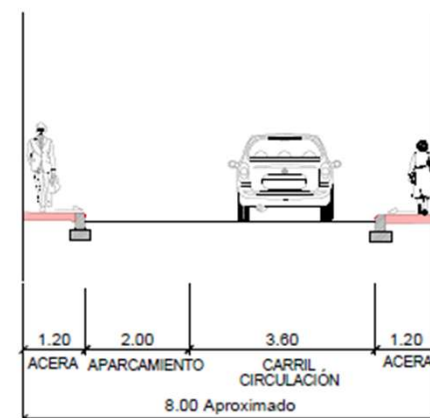
SECCIÓN D-D' TRAMO CL ALFÉREZ DÍAZ SANCHÍS
