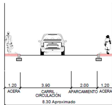
SECCIÓN C-C' TRAMO CL TENIENTE AGUADO
