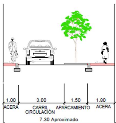
SECCIÓN A-A' TRAMO CL SARGENTO DEL RÍO
