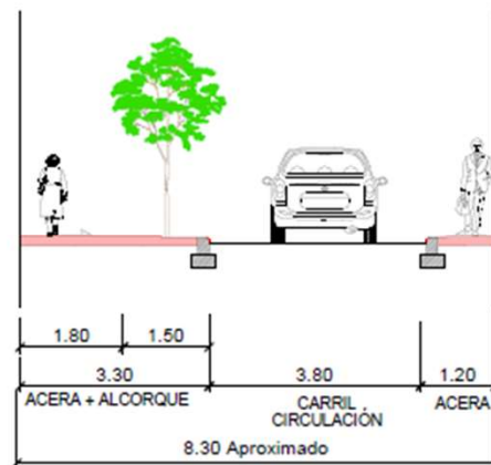
SECCIÓN C-C' TRAMO CL TENIENTE AGUADO
