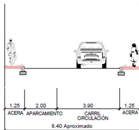
SECCIÓN B-B' TRAMO CL MAESTRO CABALLERO
