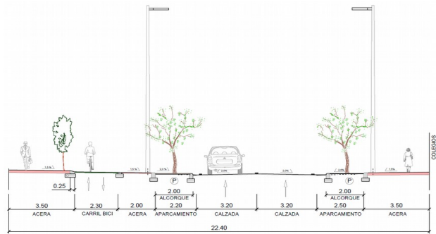
SECCIÓN TIPO A-A'
