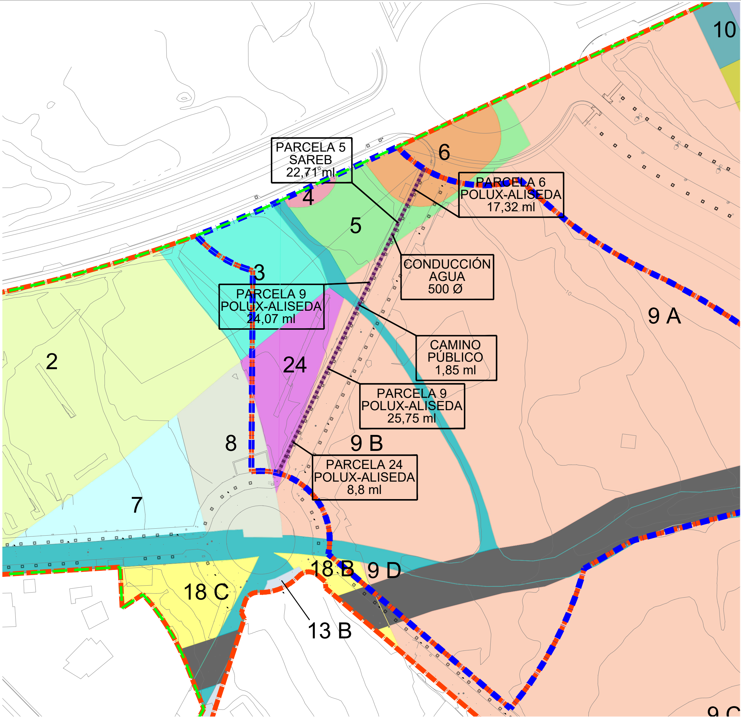
CONDICIONES DE CONEXIÓN: PASO DE INSTALACIÓN DE AGUA POTABLE EXISTENTE
