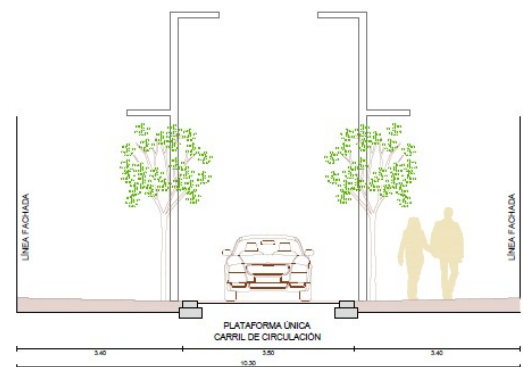
SECCIÓN 1-1' URBANIZACIÓN EL PALMERAL ESTADO REFORMADO
