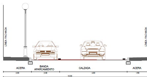
SECCIÓN 1-1' URBANIZACIÓN EL PALMERAL ESTADO ACTUAL
