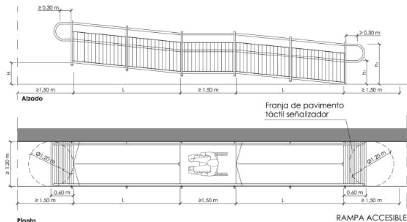
Esquema de rampa accesible.
