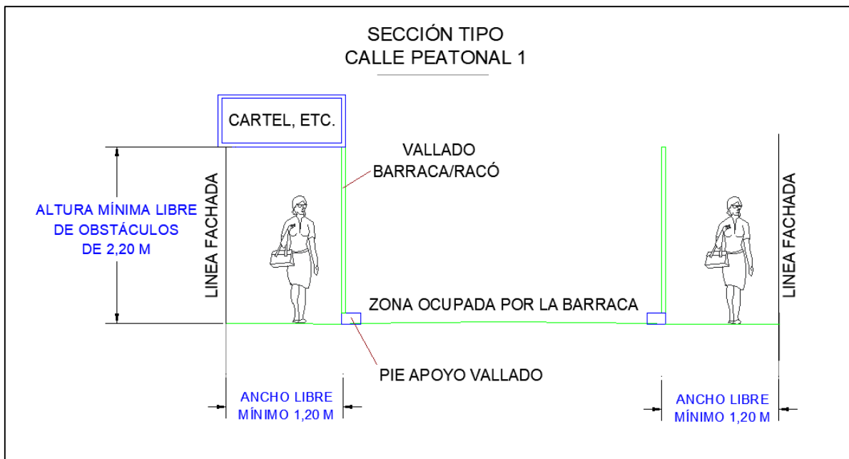
Croquis sección ocupación calle peatonal con franjas a ambos lados.
