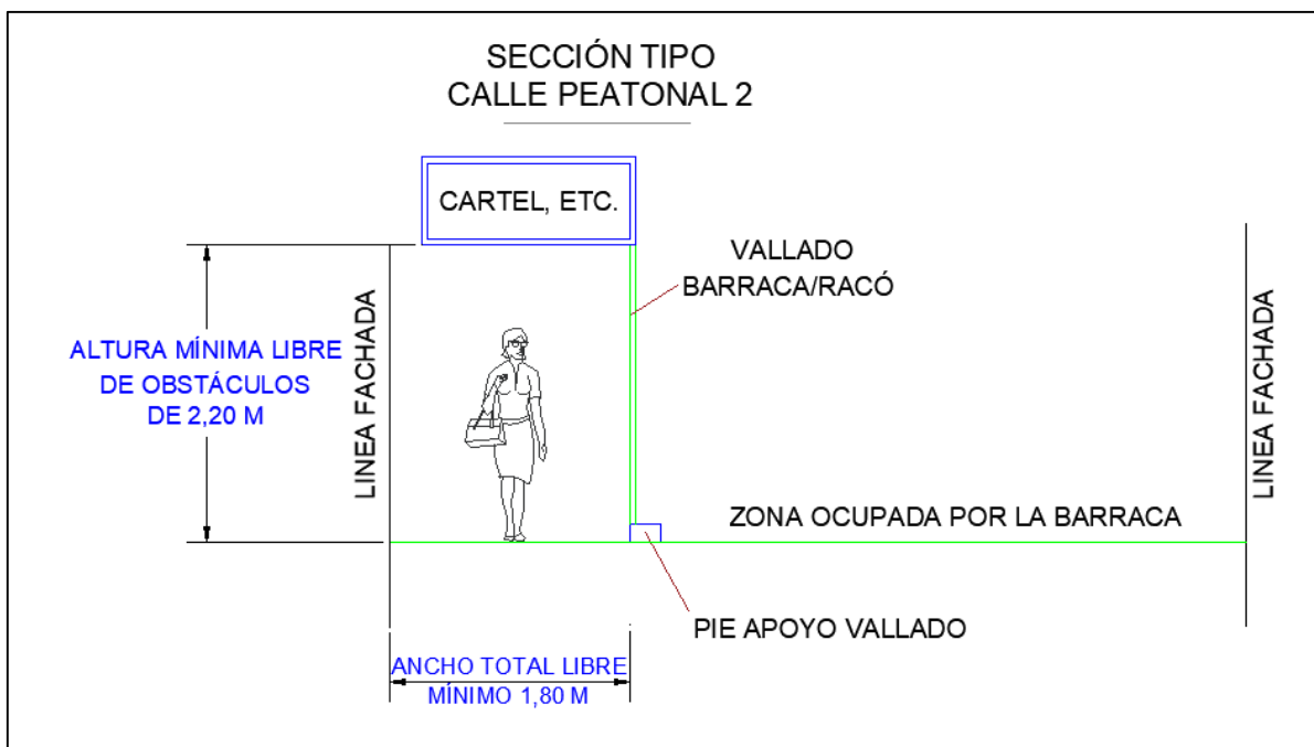
Croquis sección ocupación calle peatonal con franja un lado.
