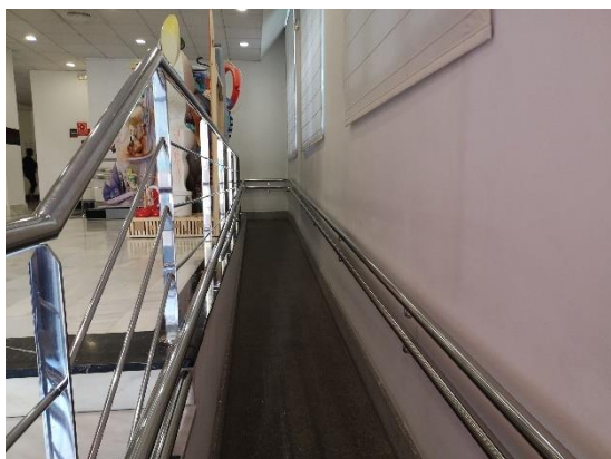
Doble pasamanos a ambos lados de rampa.
