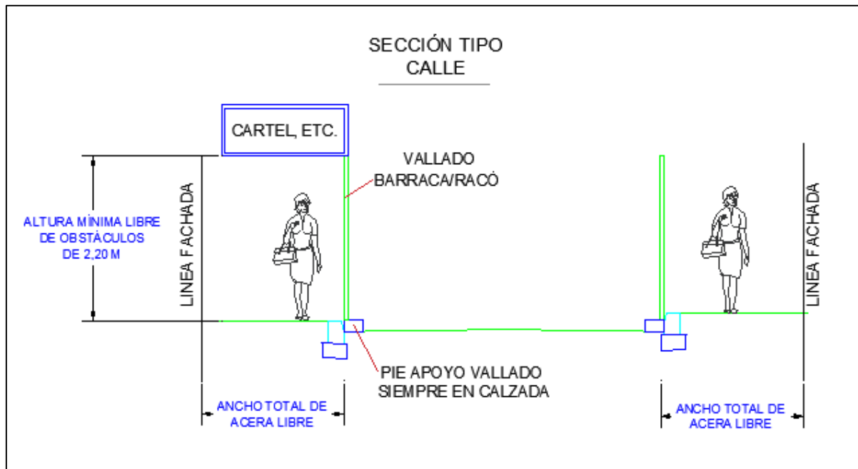
Croquis sección ocupación barraca/racó (caso general).
