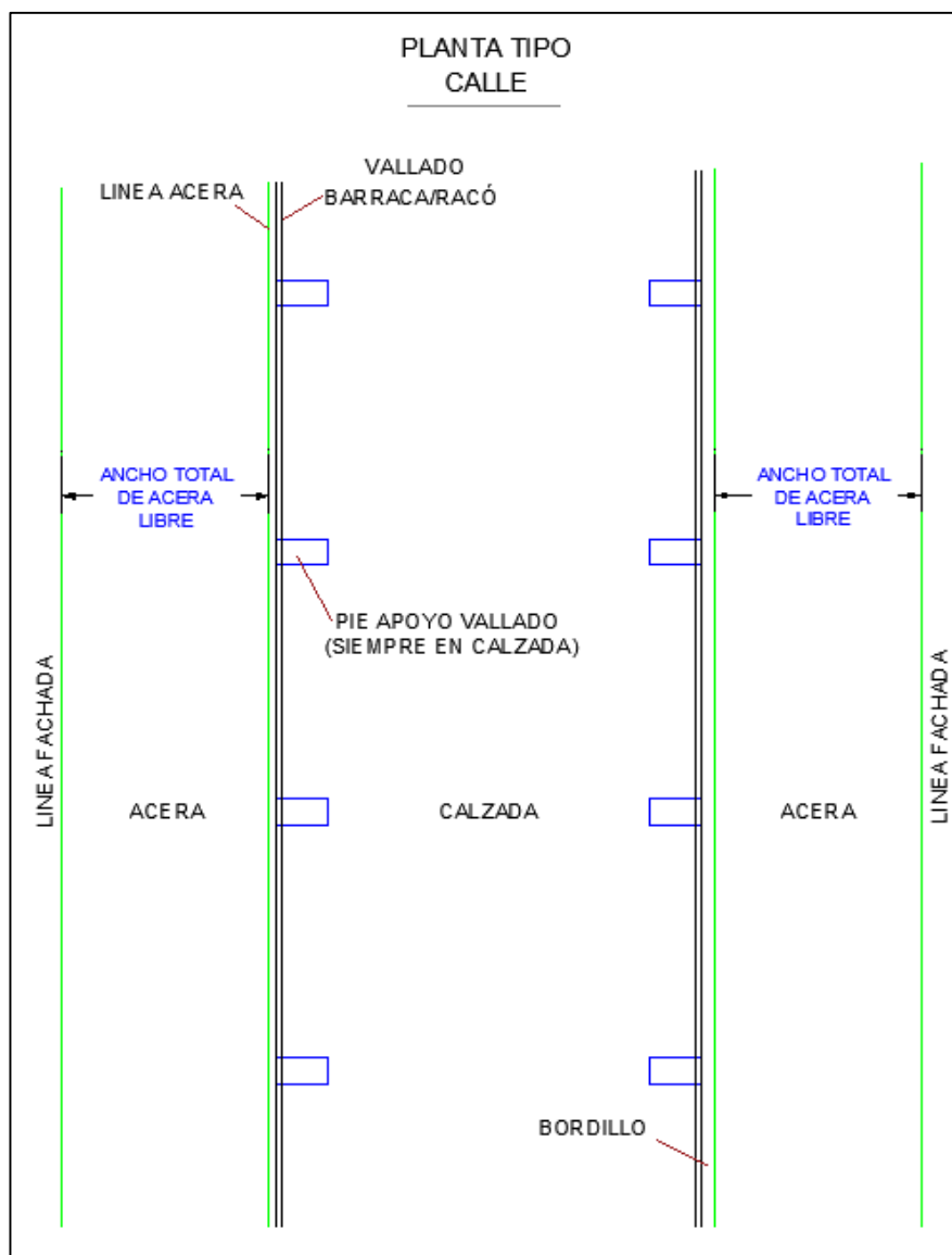
Croquis planta ocupación barraca/racó (caso general).
