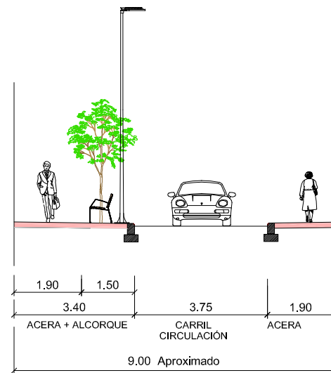
SECCIÓN A-A' - CL GENERAL ALDAVE (TRAMO CL CREVILLENTE-CL OLOZAGA)
