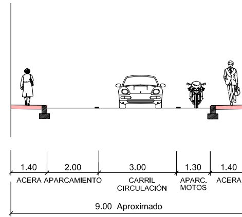
SECCIÓN B-B' - CL GENERAL ALDAVE (TRAMO CL OLOZAGA-CL DAGNIOL)
