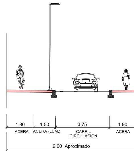
SECCIÓN B-B' - CL GENERAL ALDAVE (TRAMO CLOLOZAGA-CL DAGNIOL)
