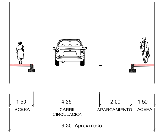
SECCIÓN D-D' - CL OLOZAGA (TRAMO CL ALCALÁ GALIANO-PZ CASTELLÓN)
