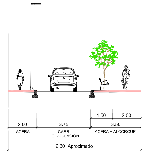
SECCIÓN D-D' - CL OLOZAGA (TRAMO CL ALCALÁ GALIANO-PZ CASTELLÓN)
