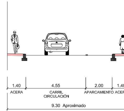
SECCIÓN C-C' - CL OLOZAGA (TRAMO AVDA. JIJONA-CL GRAL. ALDAVE)
