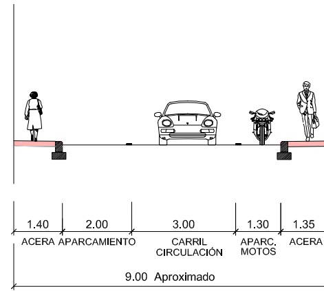
SECCIÓN A-A' - CL GENERAL ALDAVE (TRAMO CL CREVILLENTE-CL OLOZAGA)
