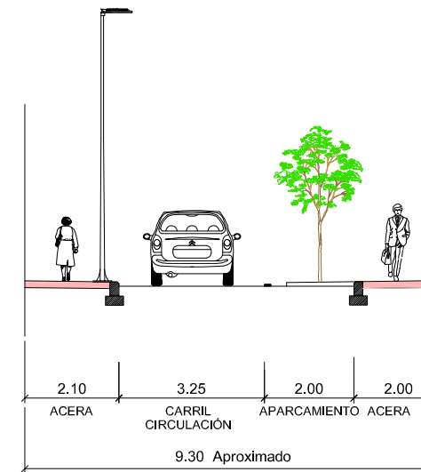
SECCIÓN C-C' - CL OLOZAGA (TRAMO AVDA JIJONA-CL GRAL.ALDAVE)
